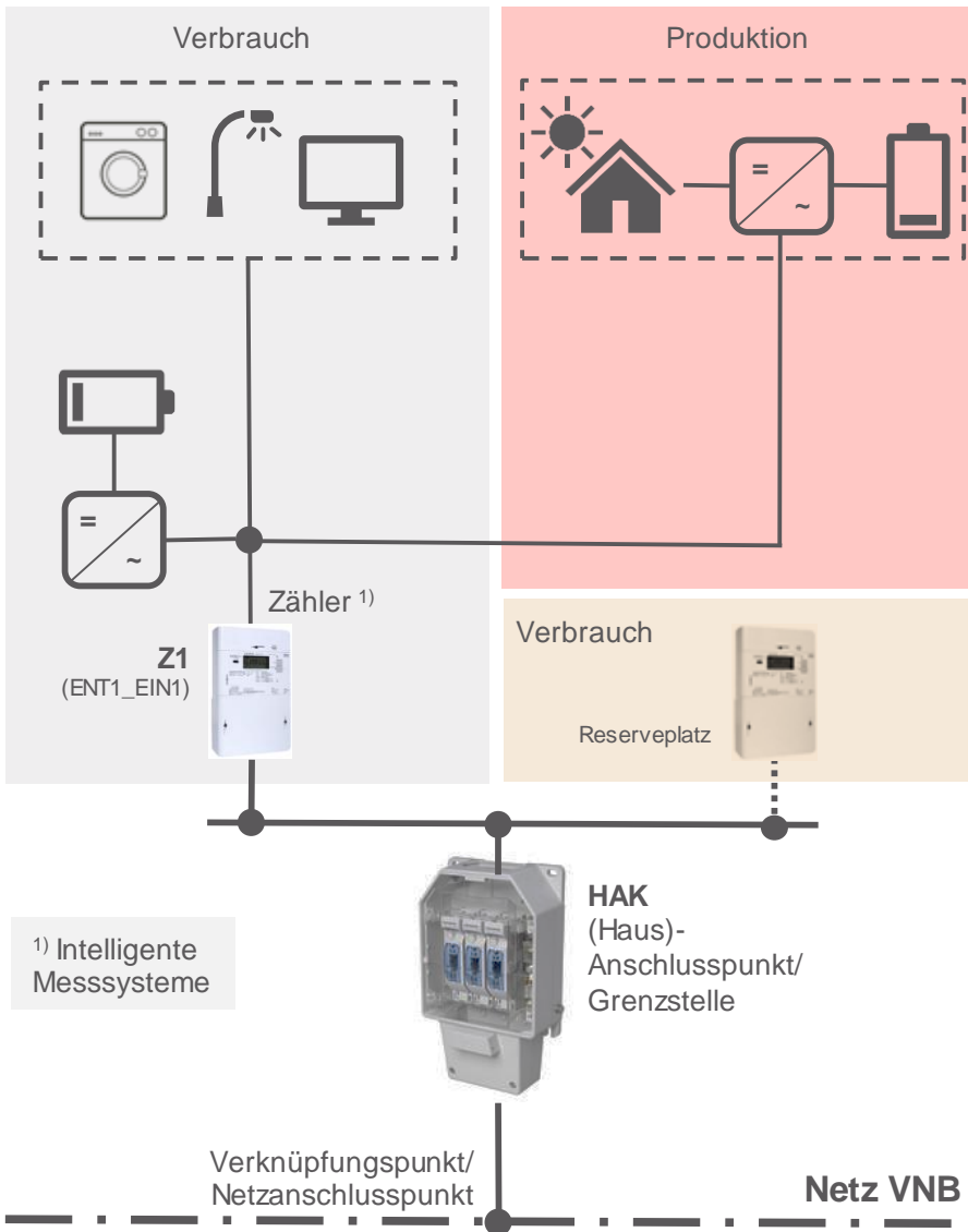
Anschlussmodell «Überschuss» (EEA < 2 kWp) «Überschuss-, Eigenverbrauchsmessung»
