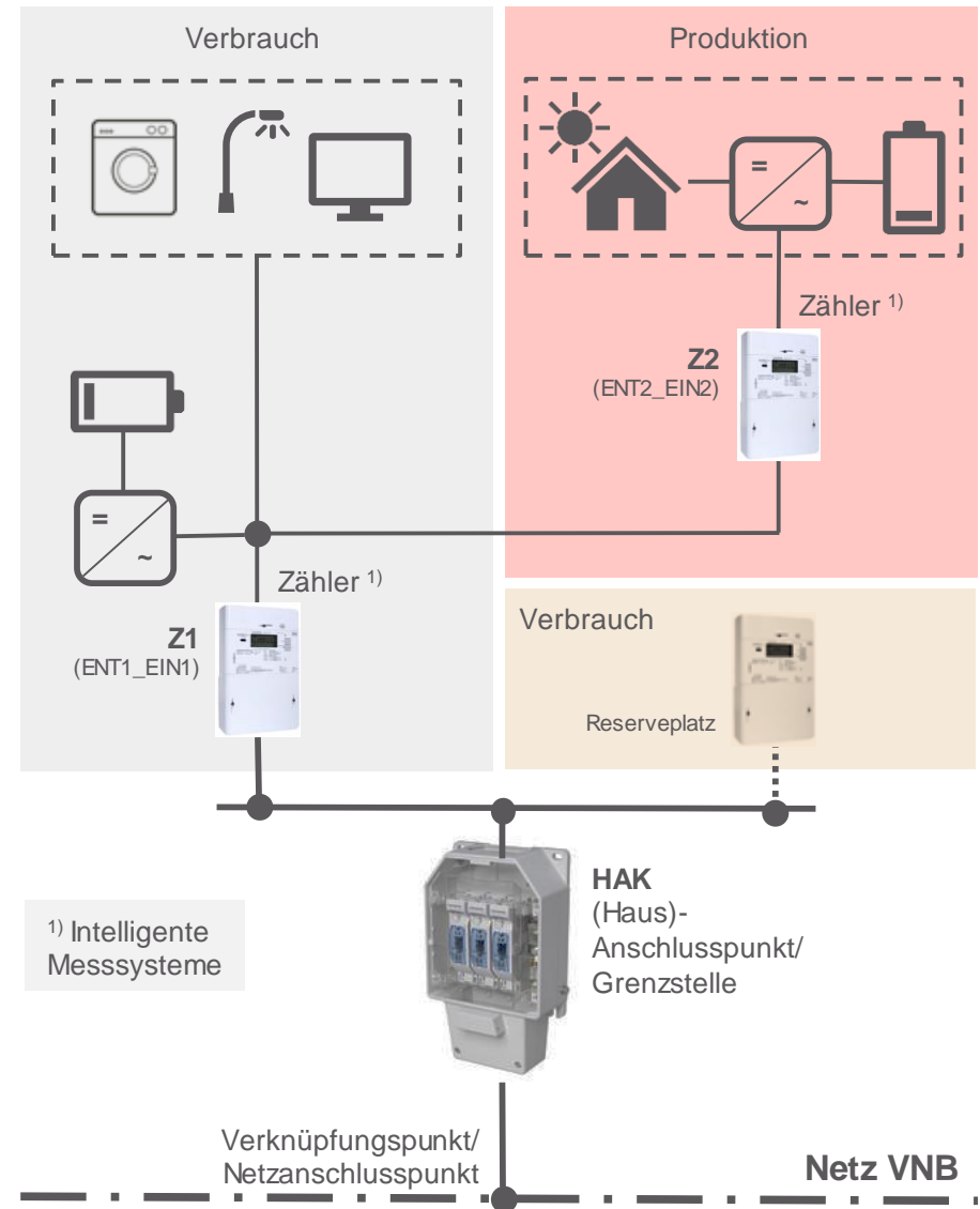
Anschlussmodell «Überschuss» (EEA ≥ 2 kWp) «Überschuss-, Eigenverbrauchsmessung»
